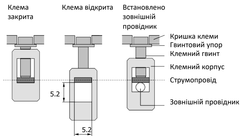
Рис. 14 E570 гвинтові зажими
