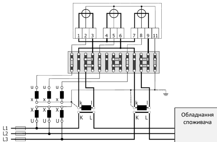
Рис. 23 Під'єднання в мережах високої напруги, 3-елементний лічильник, два ТС, ТН повна зірка
