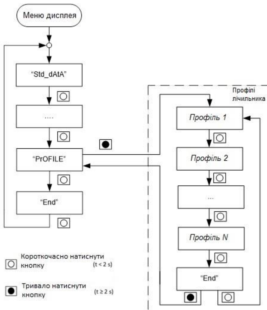
Рис. 60 Перегляд на дисплеї списку профілів
