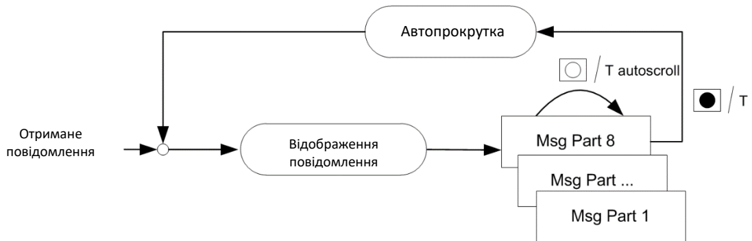
Рис. 57 Автопрокрутка при отриманні короткого повідомлення
