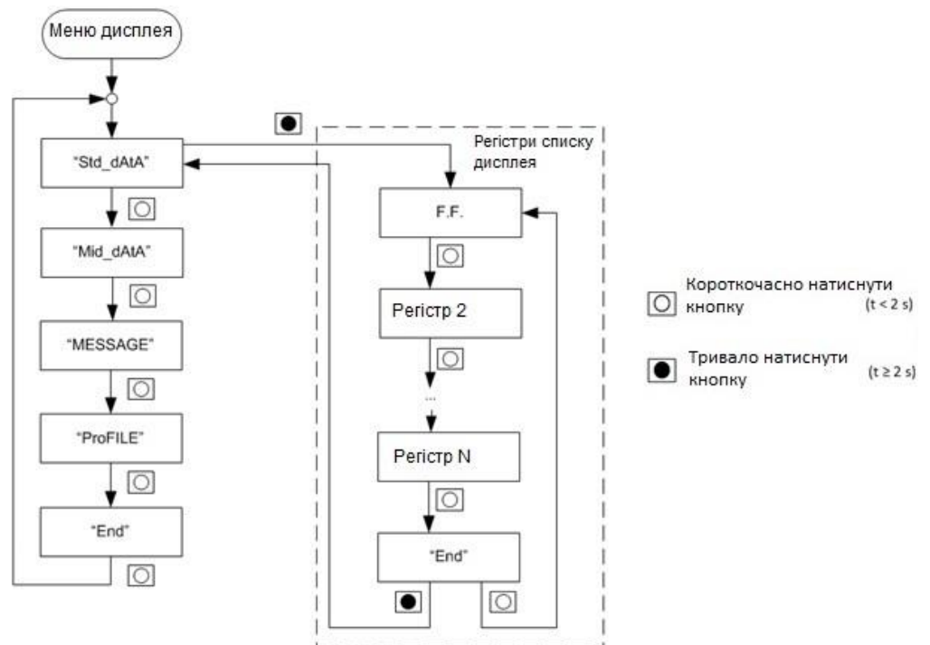
Рис. 58 Меню дисплея
