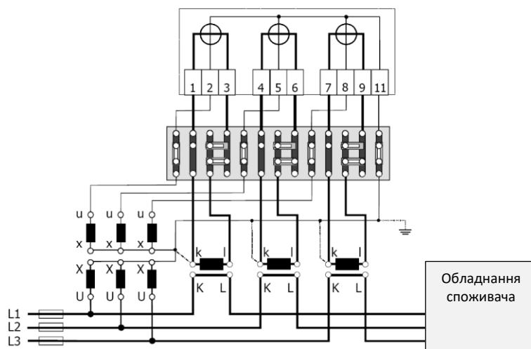
Рис. 24 Під'єднання в мережах високої напруги, три ТС, ТН повна зірка
