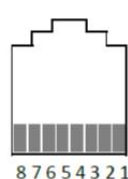
Рис. 44 Інтерфейс RS-232 модуля E57C (1 RJ45 розетка)
