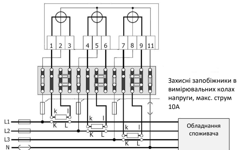
Рис. 19 М-комплекція, три ТС
