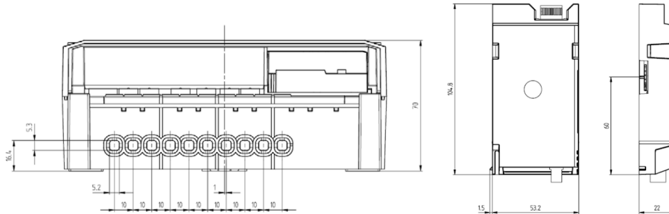
Рис. 12 Розміри колодки затискачів лічильника E570 та комунікаційного модуля E57C.
