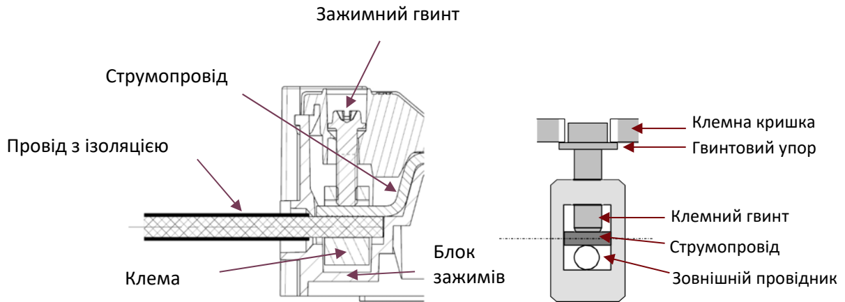
Рис. 33 Підключення лічильника
