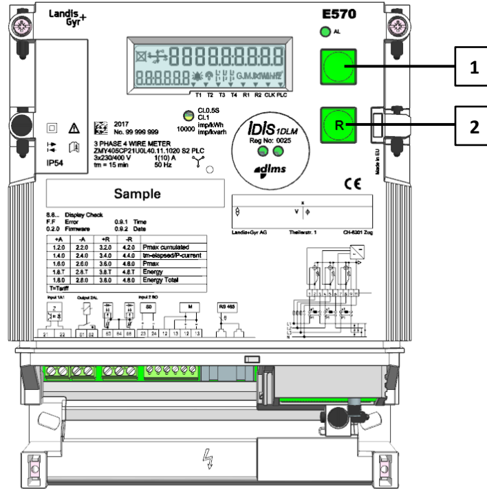
Рис. 8 Елементи управління
